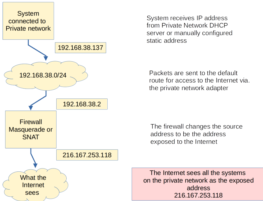
図 32.3: SNAT ないしマスカレードの例
