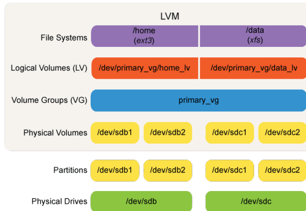
図 25.1: LVM のコンポーネント
