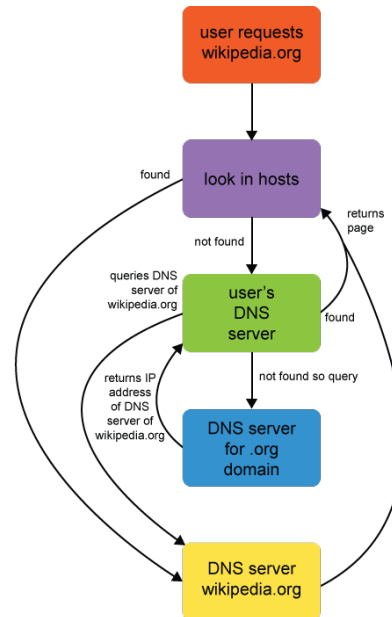
図 30.8: DNS
