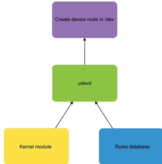
図 28.2: udev ルール
