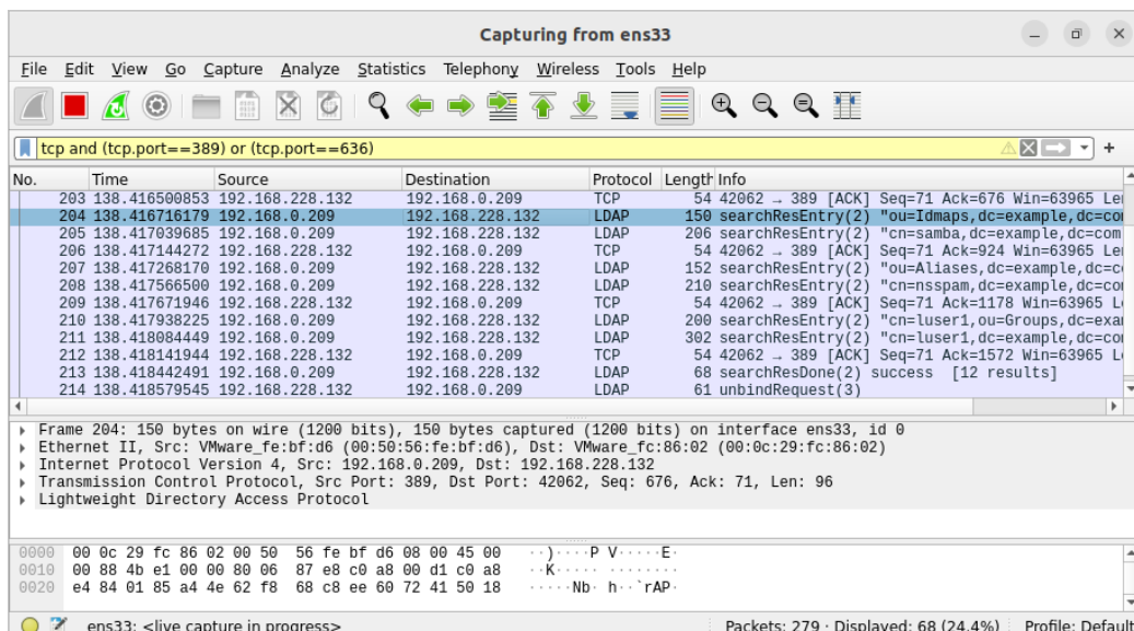
図 31.3: Wireshark による LDAP パケットのトレース
