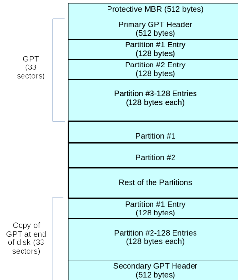
図 22.3: GPT パーティション テーブル
