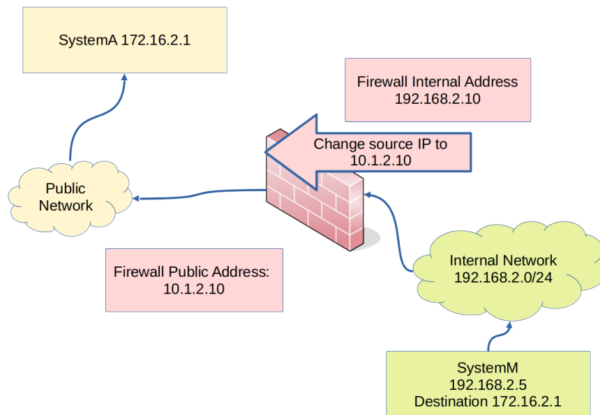
図 32.2: SNAT (ソース NAT) とマスカレード
