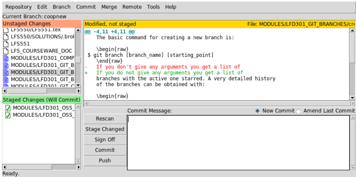
図 13.1: git gui
