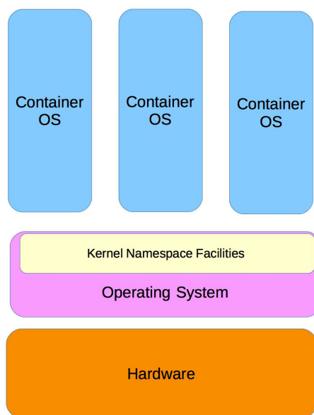
図 20.1: コンテナ
