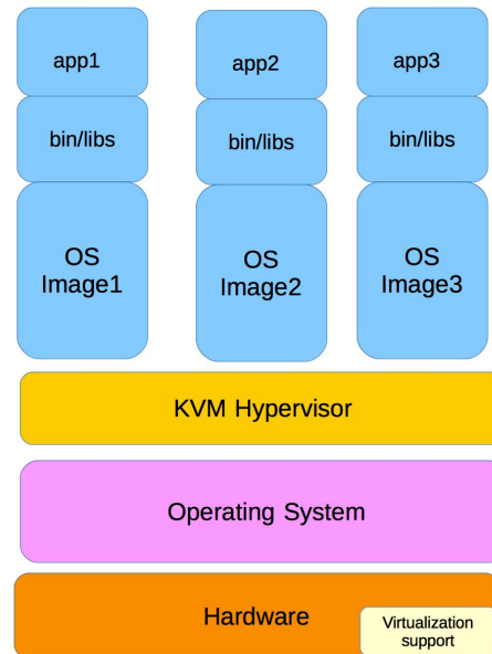
Figure 28.3: カーネル内のハイパーバイザー
