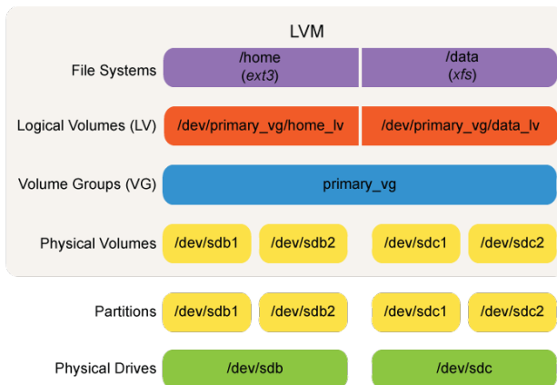
Figure 23.1: LVM のコンポーネント
