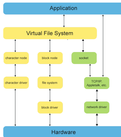
Figure 27.1: デバイスノード
