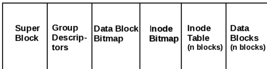
Figure 20.1: ext[3,4] ファイルシステムレイアウト
