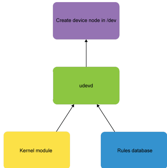
Figure 27.2: udev ルール
