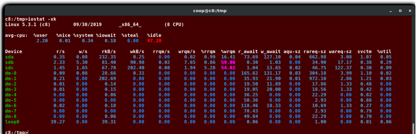
Figure 14.2: iostat の例
