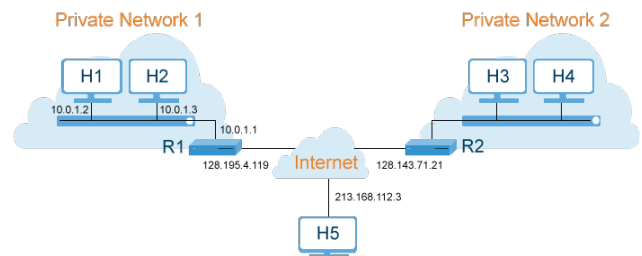
Figure 34.1: IP アドレス
